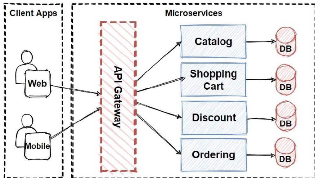
Рисунок 1.2 – Пример взаимодействия сервисов через API Gateway [3]
